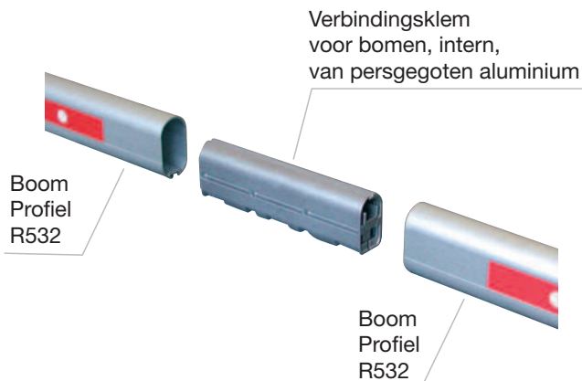
Verbindingsklem om twee boomstukken R532 te verenigen.
