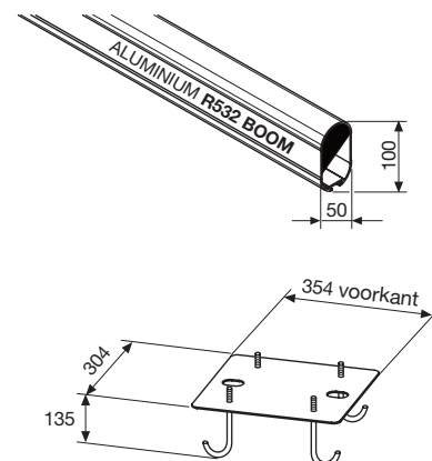
Verankeringsplaat 354x304 met ankerbouten M14x200
