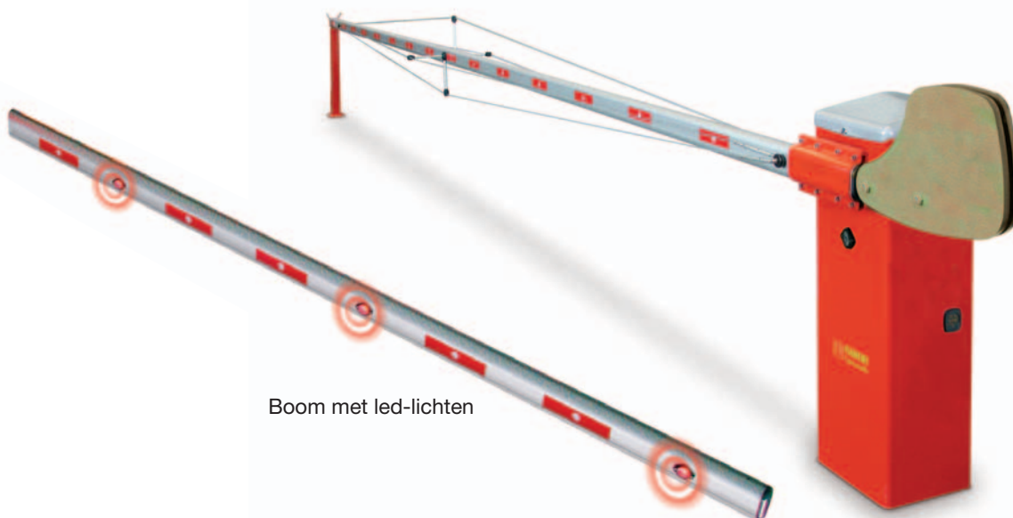
Bayt 980 rechtversie van 8,0 meter met versterkingskabels, contragewichten, gelakte kast. Ook in de inox RVS versie.
